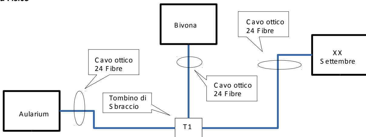
Schema Logico
