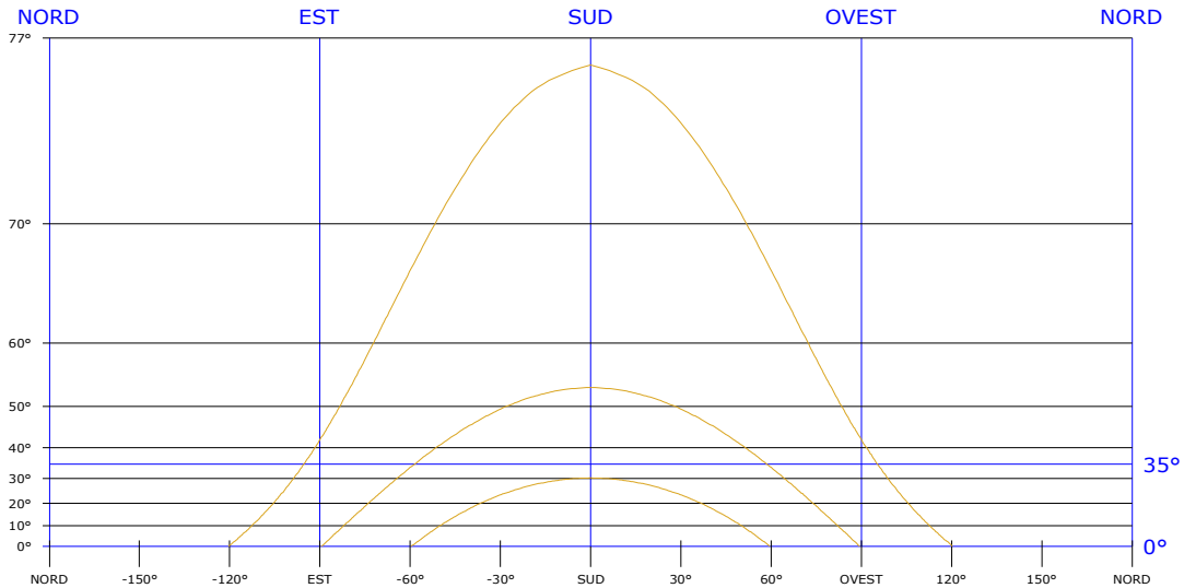
Fig. 3: Diagramma solare
