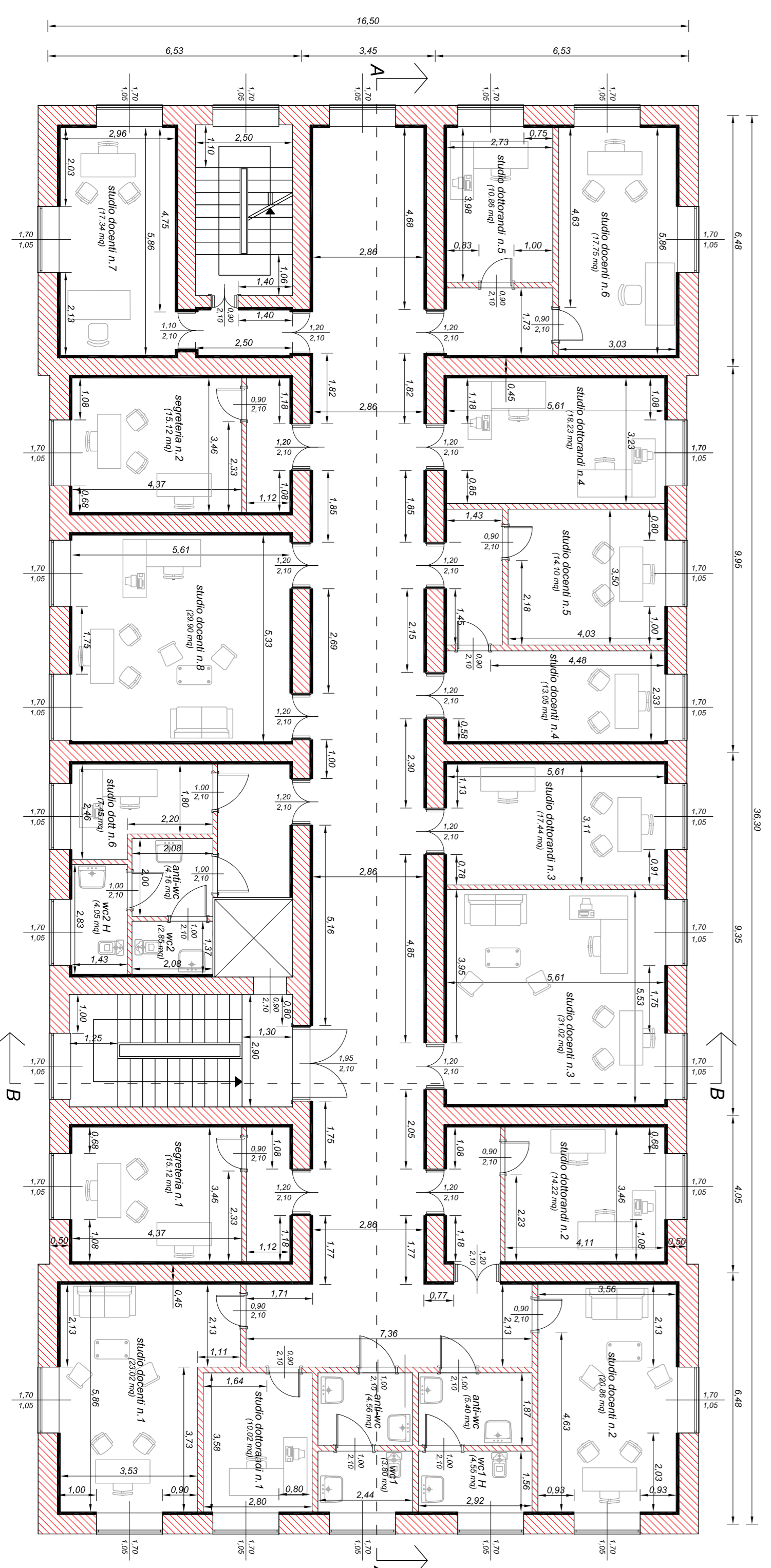
Pianta piano intermedio stato di progetto Scala (1:100)
